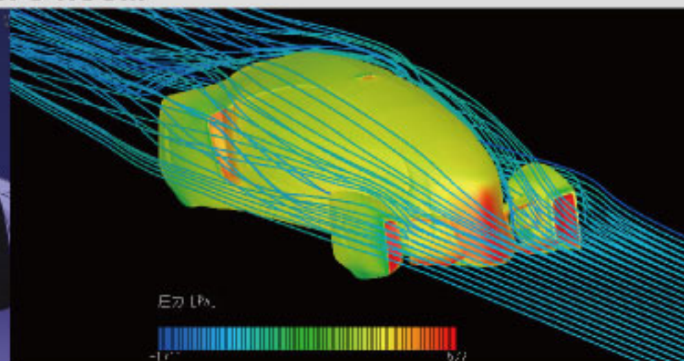
SCRYU / Tetra
