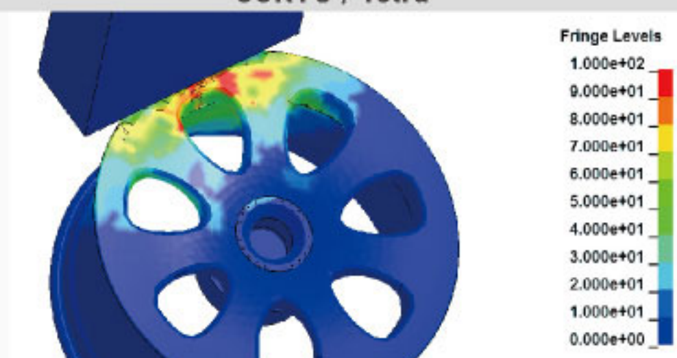
LS-DYNA
